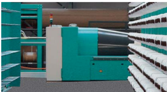
2 Creel operation 2 Gatter Betrieb
