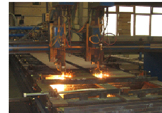
Brennschneiden
